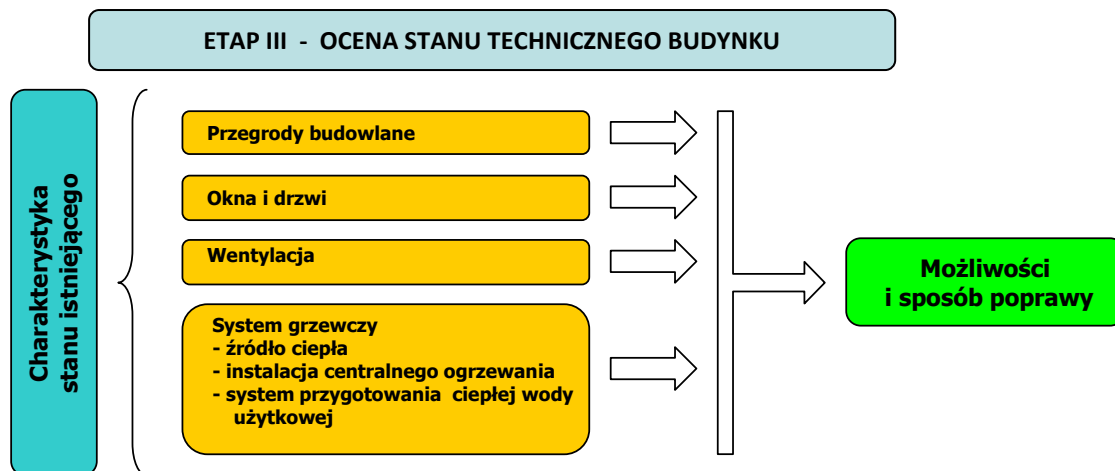
Rys. 4 Schemat przeprowadzania oceny stanu technicznego budynku
